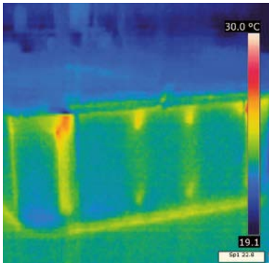
Test úniku tepla se systémem Nordic Insulation
